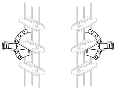
comando alavanca
