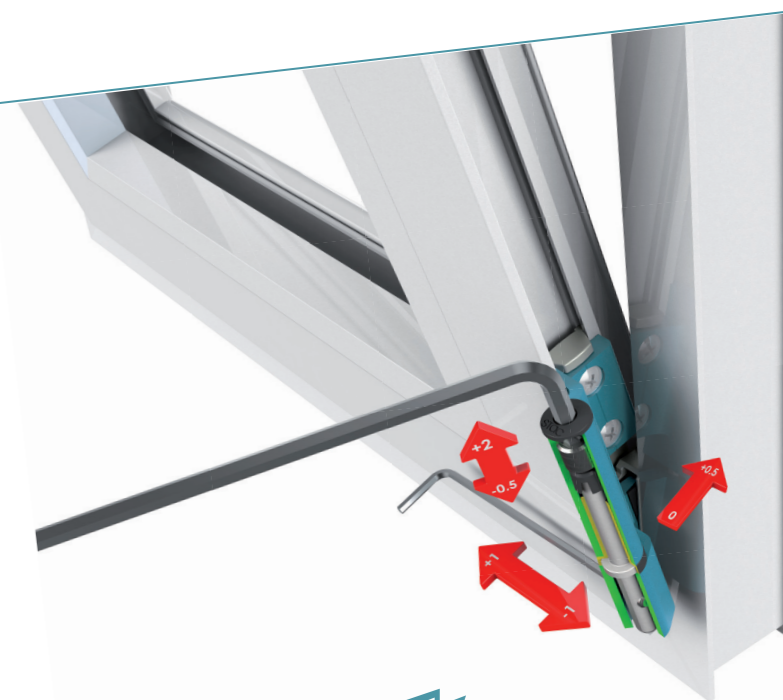
BISAGRA INFERIOR
