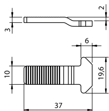
2030 GRAMPO INOX emb. 50 un.
