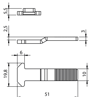
09769 PEÇA ZAMAK MICRO DE CORRER emb. 50 un.
