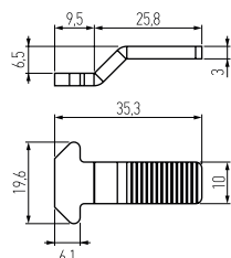
4307G PEÇA ZAMAK PERIMETRAL emb. 50 un.
