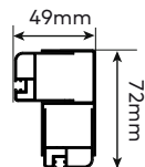
Perfil canto Corner profile.
